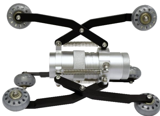
Type-B Skid
